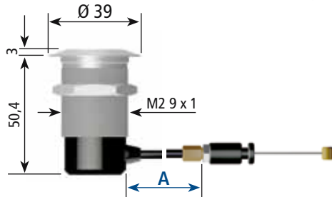
Protruding push-button with axial bowden cable exit Hohe Taste mit axialem Bowdenzugausgang
